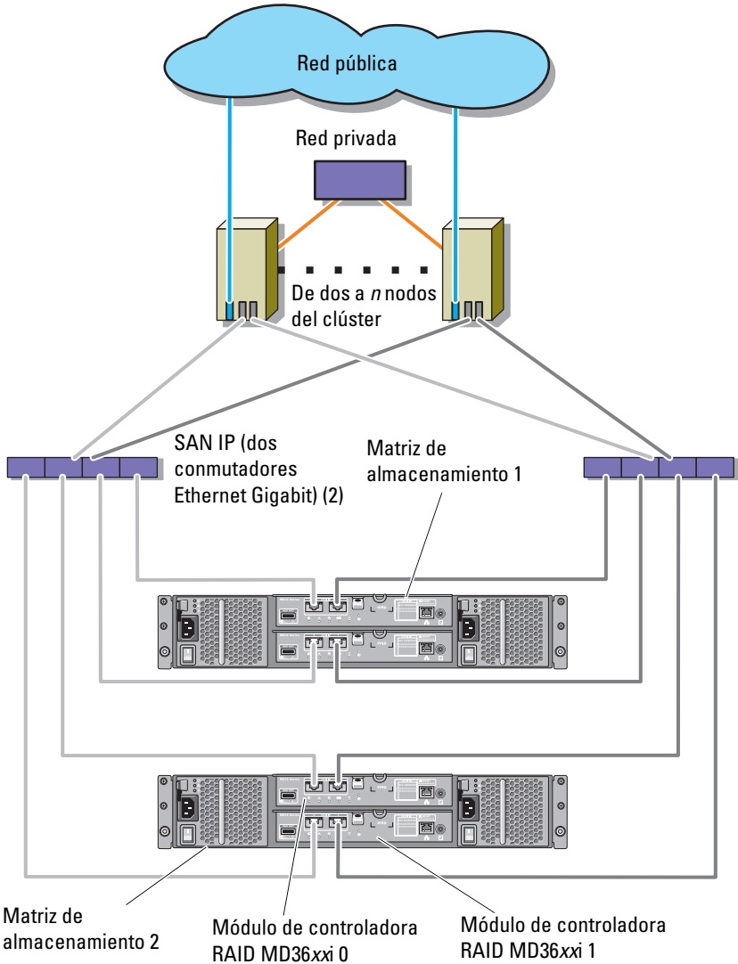
Ilustración 2-5. Configuración de clúster de conexión mediante red con varias matrices de almacenamiento
