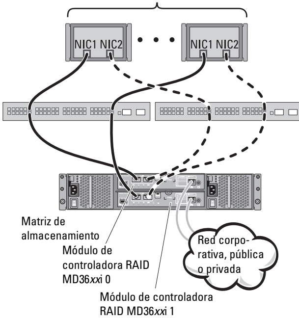
Ilustración 1-2. Configuración de clúster de conexión mediante red redundante
