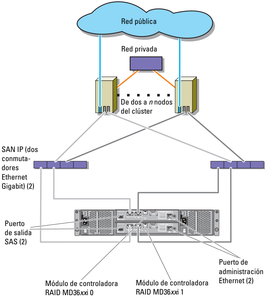
Ilustración 2-4. Configuración de clúster de conexión mediante red
