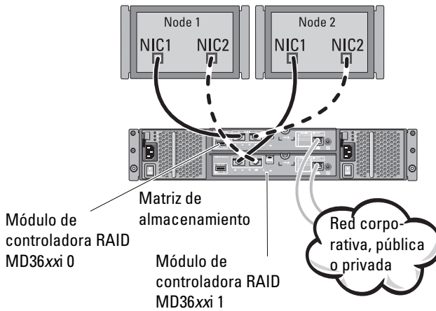
Ilustración 1-1. Configuración de clúster de conexión directa
